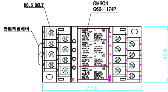
투명PC커버 개방시
